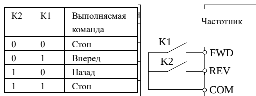
Рис.6-13 Двухпроводной режим управления 1
