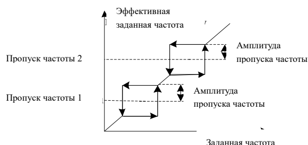
Рис. 6-5 Пропуск частот
