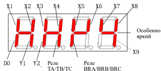
Рис. 6-28 Схема отображения текущего состояния статуса клемм
