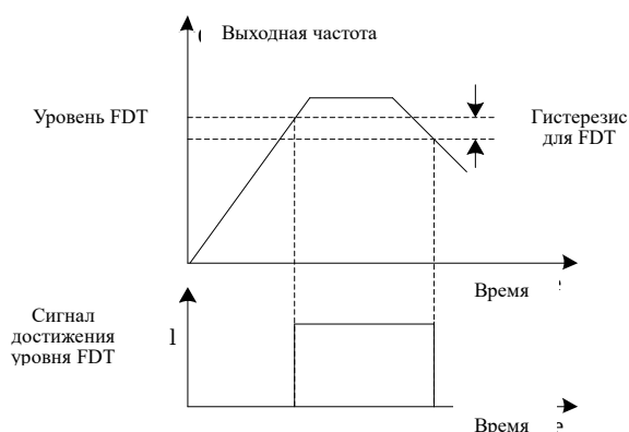
Рис. 6-21 Уровень FDT и схема задержки
