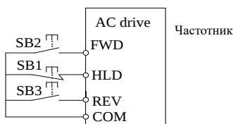
Рис.6-15 Трехпроводной режим управления 1
