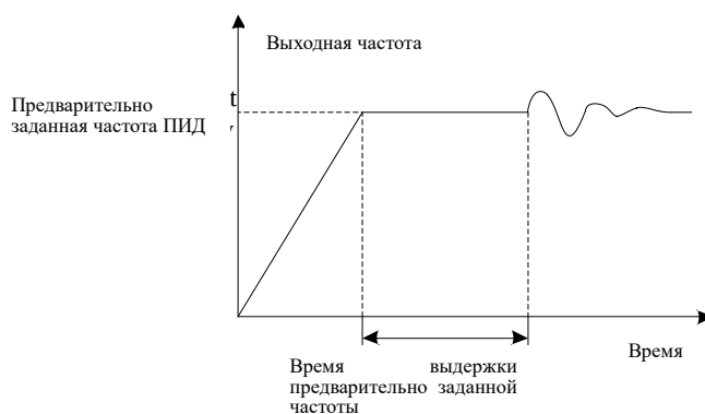
Рис. 6-24 Предварительно заданная частота и время выдержки предварительно заданной частоты ПИД
