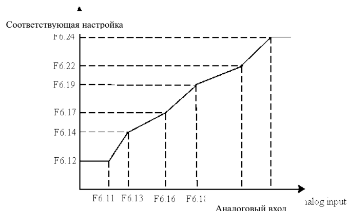
Рис. 6-17 Нелинейная кривая аналогового входа
