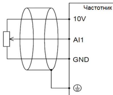
Рис. 3-14 Подключение аналоговых входов
