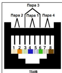
Рис. 3-15 Стандартный T568B
