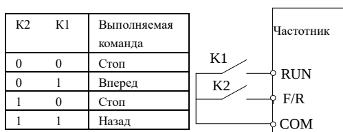
Рис. 6-14 Двухпроводной режим управления 2
