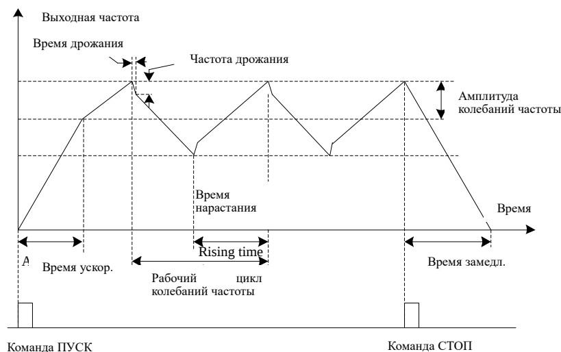
Рис. 6-26 Схема изображения колебаний частоты
