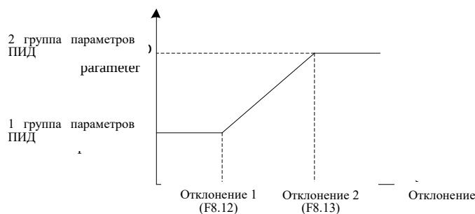
Рис. 6-23 Переключение параметров ПИД
