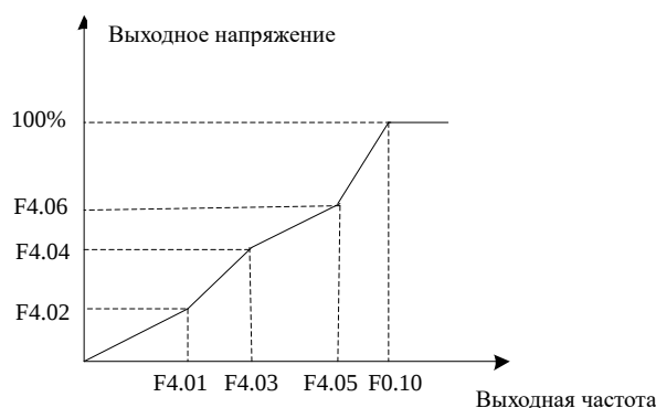
Рис.6-9 Кривая зависимости напряжения от частоты, определяемая пользователем
