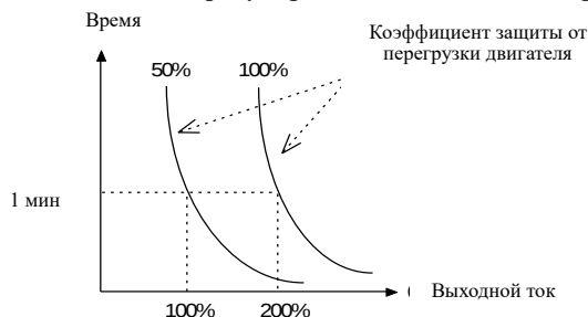
Рис. 6-27 Кривая защиты двигателя от перегрузки
