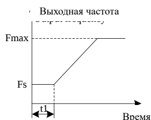
Рис.6-3 Пусковая частота и время выдержки пусковой частоты
