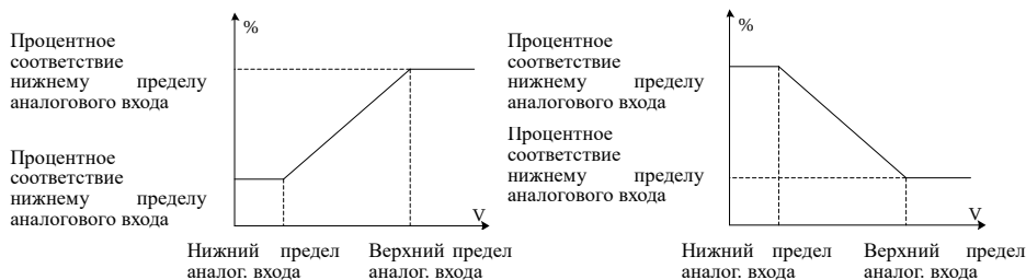
Рис. 6-18 Линейная кривая аналогового входа
