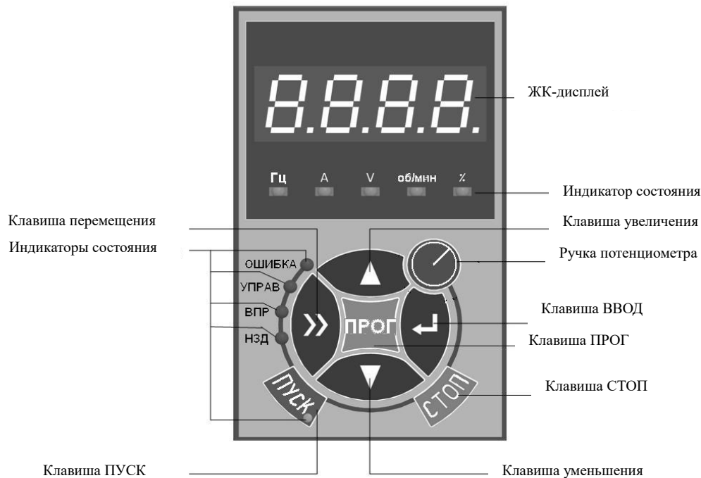
Рис. 4-1 Рисунок панели управления
