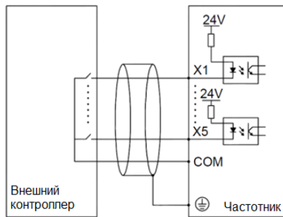
Рис. 3-10 Схема подключения цепи управления
