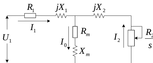
Рис. 6-12 Эквивалентная схема асинхронного двигателя
