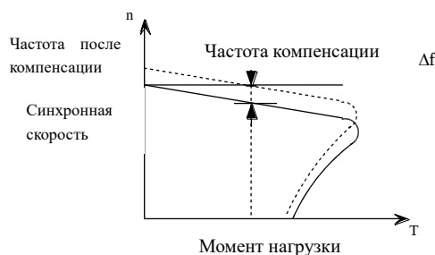
Рис. 6-11 Автоматическая компенсация скольжения
