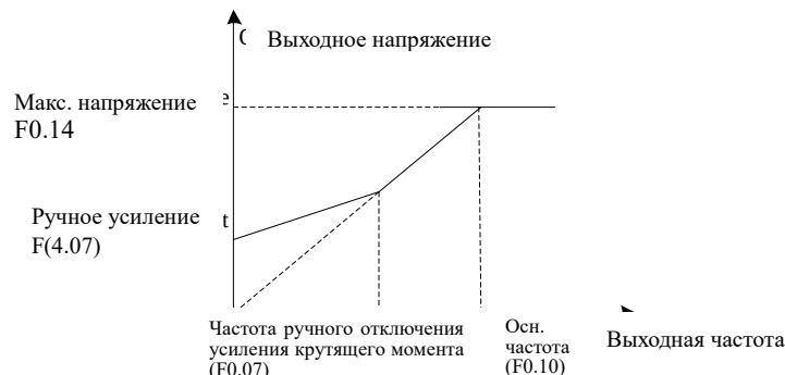
Рис.6-10 Схема усиления крутящего момента
