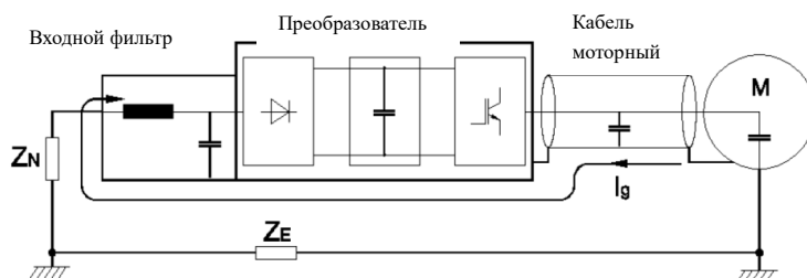
Рис. 3-6 Меры по борьбе с помехами
