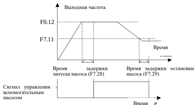
Рис. 6-22 Сигнал управления вспомогательным насосом для постоянной подачи воды под давлением
