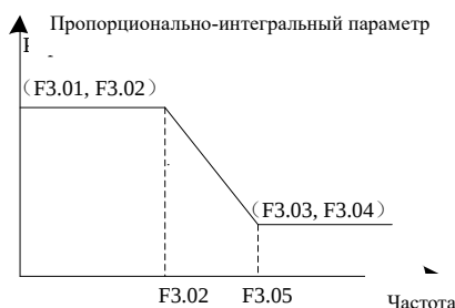
Рис. 6-7 Схема пропорционально-интегральных параметров контура скорости
