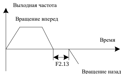
Рис. 6-6 Переключение вперед/назад
