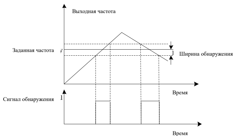
Рис.6-20 Схема обнаружения FAR
