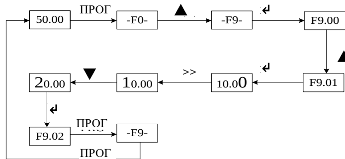
Рис.4-3 Пример работы 3 уровней меню
