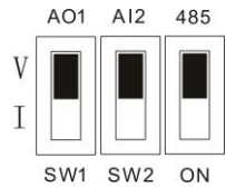
Рис. 3-17 Настройка двухпозиционного переключателя
