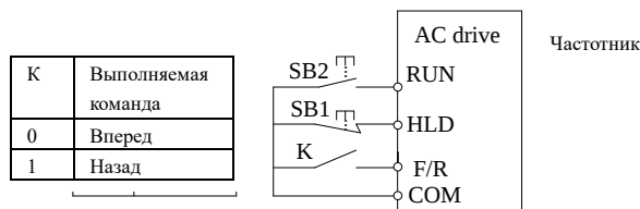
Рис.6-16 Трехпроводной режим управления 2
