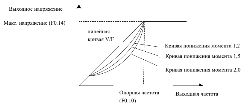
Рис. 6-8 Кривая понижения крутящего момента
