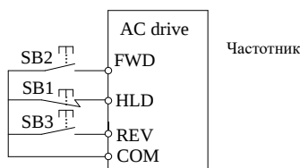
Рис.6-15 Трехпроводной режим управления 1
