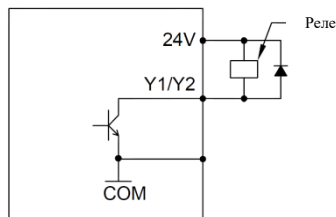
Рис. 3-16 Способ подключения внутреннего источника питания +24 В
