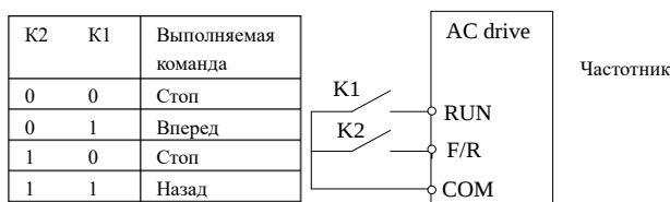
Рис. 6-14 Двухпроводной режим управления 2
