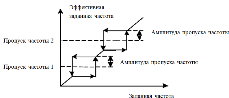
Рис. 6-5 Пропуск частот
