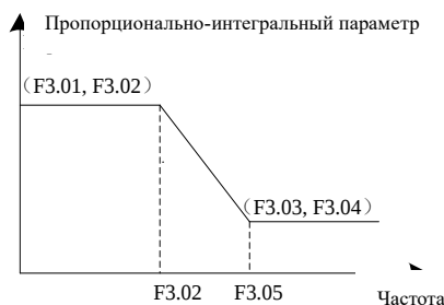
Рис. 6-7 Схема пропорционально-интегральных параметров контура скорости
