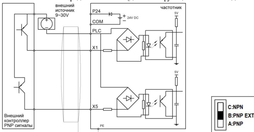
Рис. 3-14 Стандартный способ подключения PNP с внешним источником питания 24VDC
