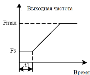
Рис.6-3 Пусковая частота и время выдержки пусковой частоты
