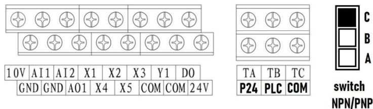
Рис. 3-10 Расположение клемм цепи управления для версии B2_0102/0302
