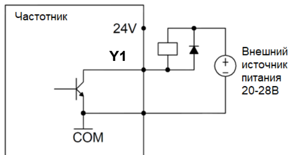
Рис.3-17 Способ подключения внешнего источника питания
