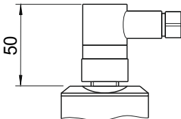
Версия электросоединения с разъемом M12x4pin
