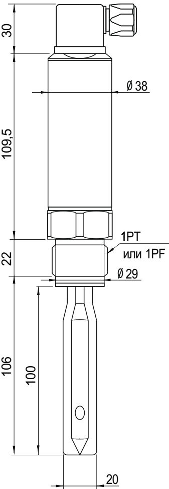
Версия с резьбой 1" и разъемом DIN 43650
