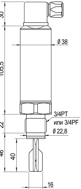
Версия с резьбой 3/4" и разъемом DIN 43650
