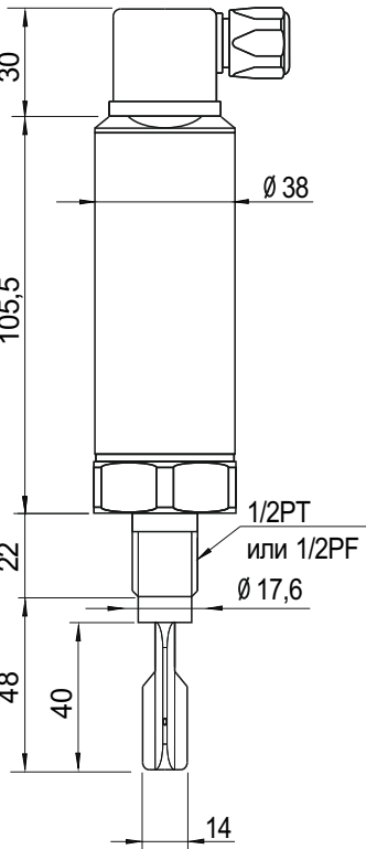
Версия с резьбой 1/2" и разъемом DIN 43650
